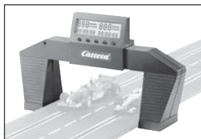
71590 Elektronischer Rundenzähler · Electronical lap counter · Compte-tours électronique · Cuentavueltas electrónico · Contador electrónico de voltas
