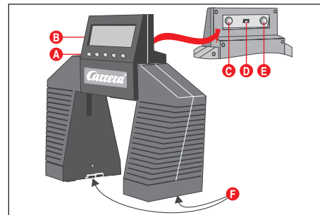
1 Elektronischer Rundenzähler
